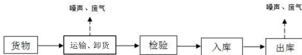
图 2-3 项目营运期流程及产污节点图
