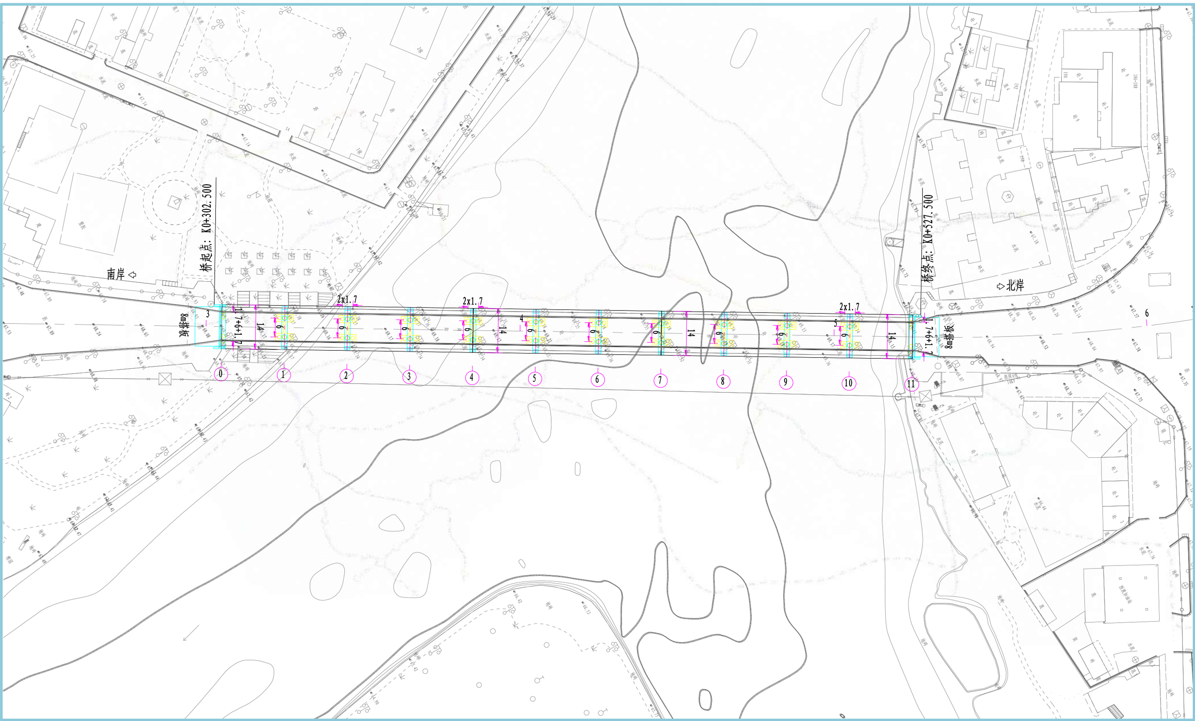
衡阳县向阳大桥维修加固工程建设项目规划平面图
