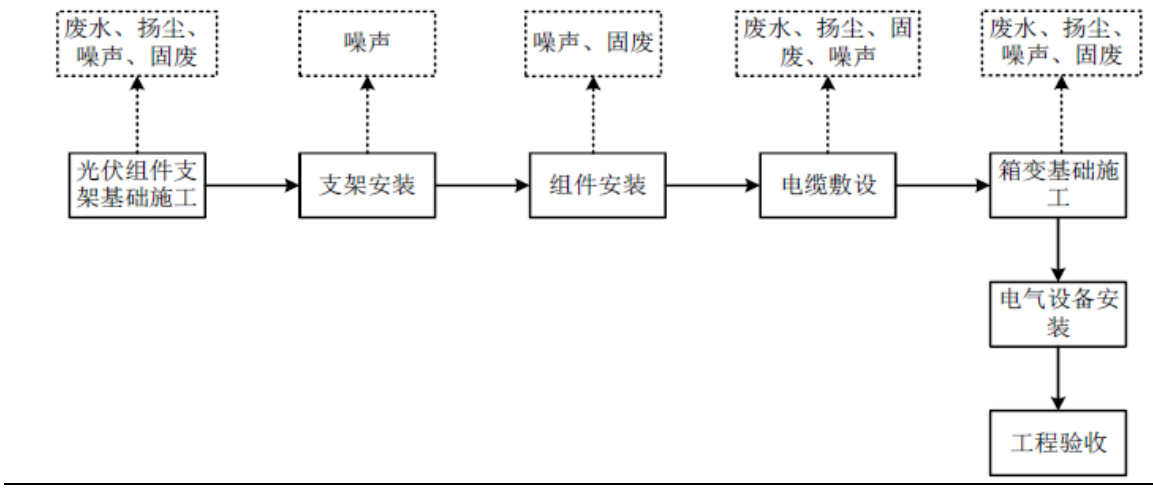
图 2-3 光伏区施工工艺及产污环节
